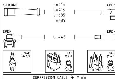
SUPPRESSION CABLE Ø 7 mm
