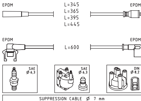
SUPPRESSION CABLE \varnothing 7 mm
