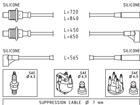
SUPPRESSION CABLE Ø 7 mm
