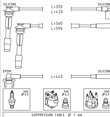
SUPPRESSION CABLE Ø 7 mm
