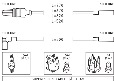
SUPPRESSION CABLE Ø 7 mm
